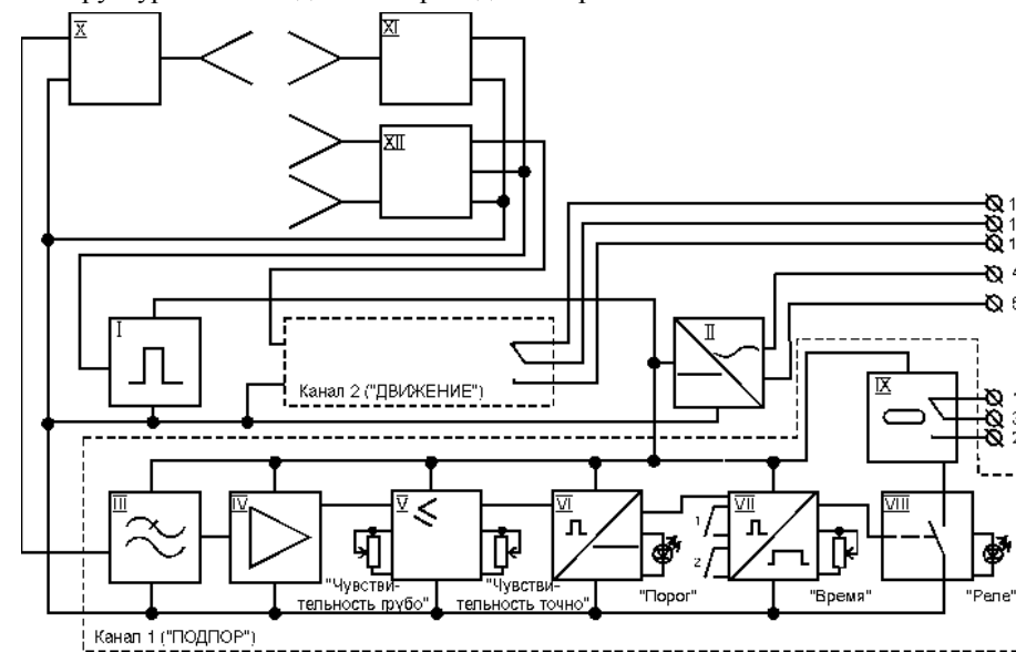
Рис. 5. Структурная схема РДПИ-02.
