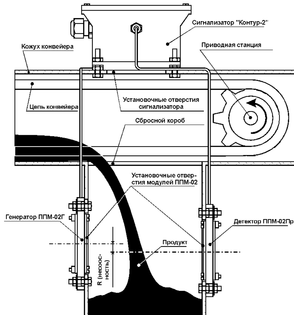
Рис.3. Монтаж датчика РДДП-02.
