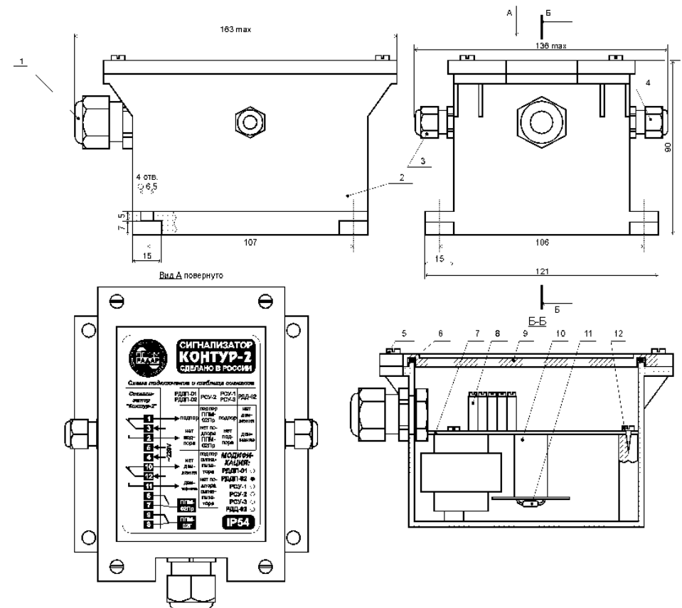
Рис. 1. Конструкция сигнализатора «Контур-2» (модификация «РДДП-02»).
